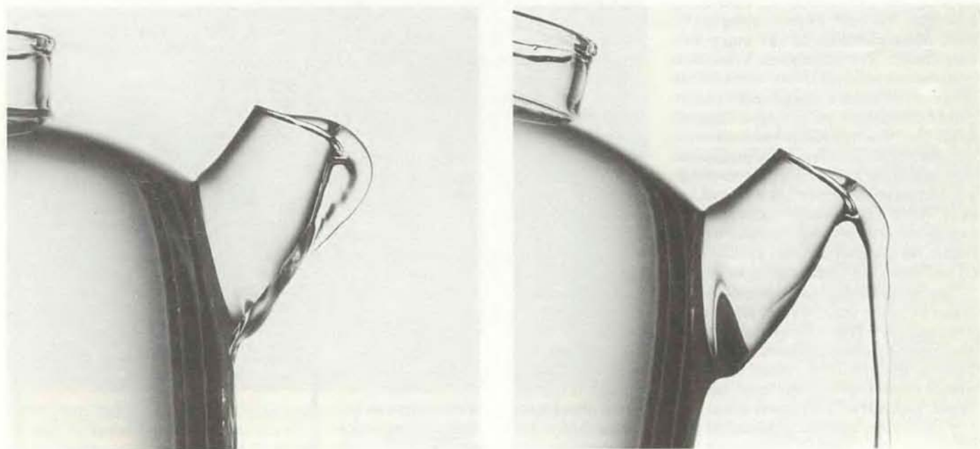
Слева — вода, текущая по носику чайника (чайниковый эффект), справа — свободная струя
