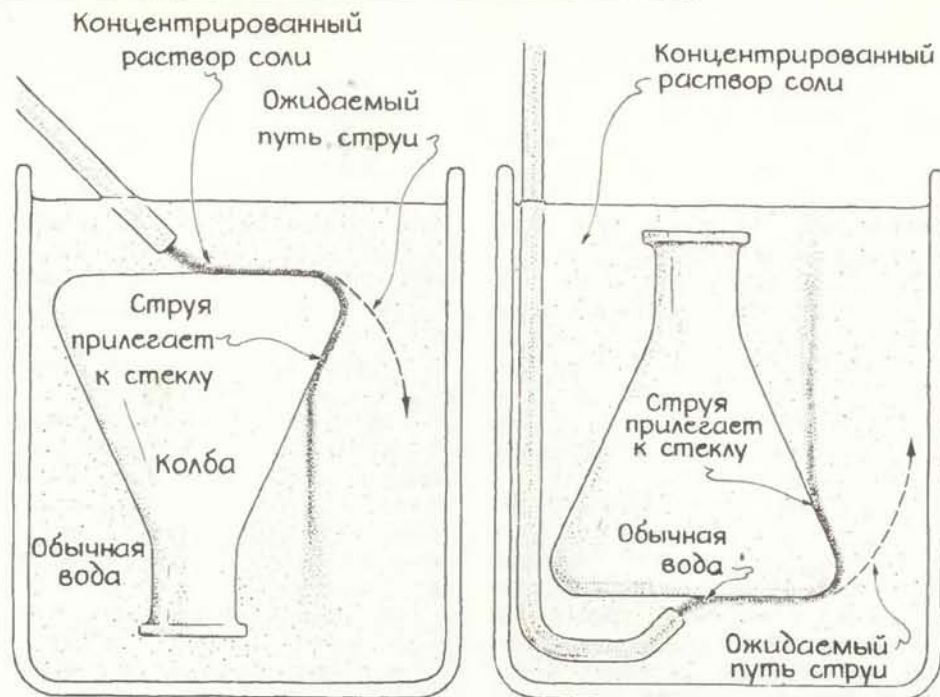
Опыты М. Рейнера с соленой и обычной водой
