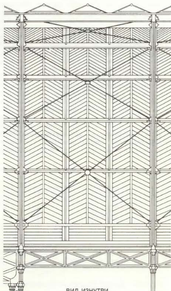
ВИД ИЗНУТРИ
