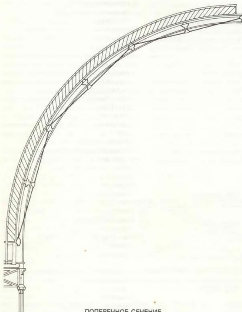
ПОПЕРЕЧНОЕ СЕЧЕНИЕ
