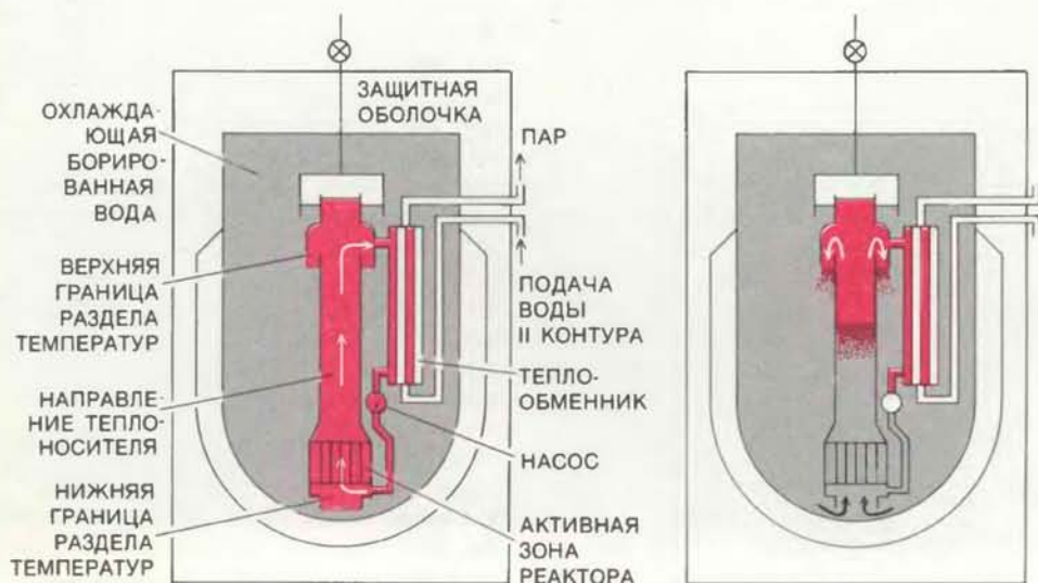
Конструкция ПСБ-реактора такова, что возможность утечки воды из активной зоны исключена; при аварии системы охлаждения активная зона заполняется раствором борной кислоты
