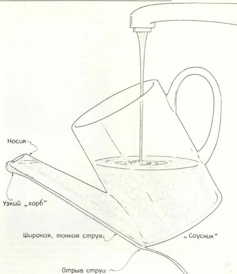
Приспособление для исследования чайникового эффекта
