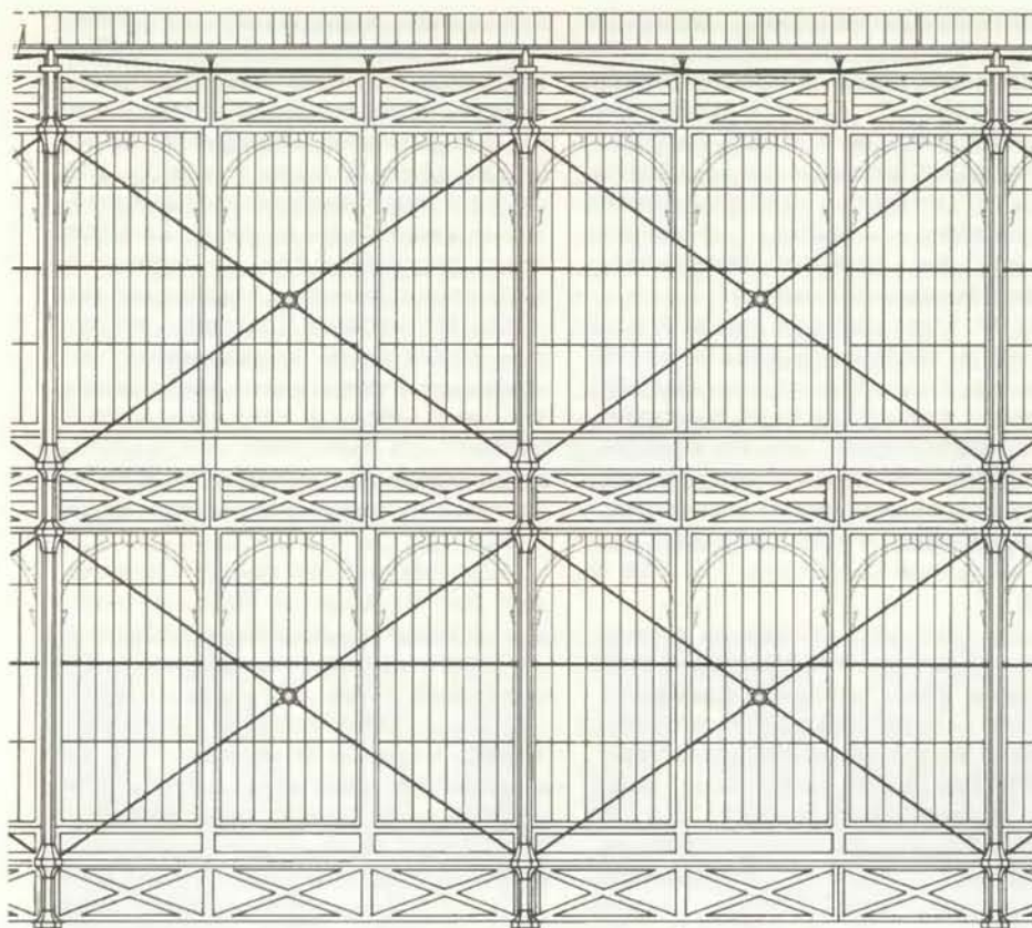
СТЕРЖНИ ИЗ КОВКОГО ЖЕЛЕЗА обеспечивали жесткость наружным стенам Хрустального дворца, не имевшего внутренних стен. Видимые снаружи и изнутри, эти стержни — стяжки придавали зданию современный вид.
