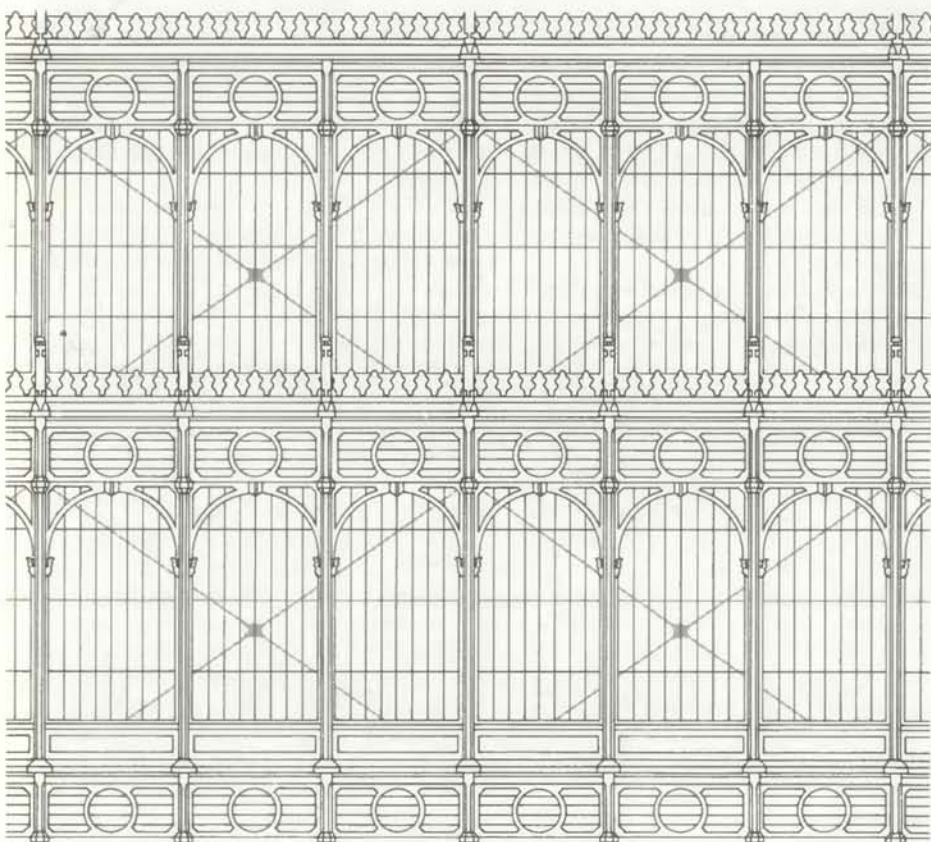
ОТВЕСНЫЕ СТЕНЫ — это еще одно новшество, введенное Пакстоном и его коллегами. Панели из стекла размером 125 × 25 см устанавливались за тонкими обрамляющими арками. Такие панели использовались для остекления как стен, так и крыши. На весь дворец потребовалось примерно 400 т стекла. Прозрачная «оболочка» Хрустального дворца послужила прототипом для многих современных зданий.
