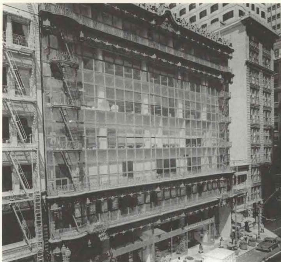
ПОЛНОСТЬЮ ЗАСТЕКЛЕННЫЙ ФАСАД здания Хэллади-билдинг, построенного в Сан-Франциско по проекту У. Полка в 1915 г. Впервые идея стеклянных стен была воплощена в Хрустальном дворце.
