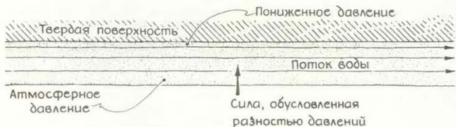
Сила, удерживающая «перевернутый» поток, согласно Дж. Келлеру
